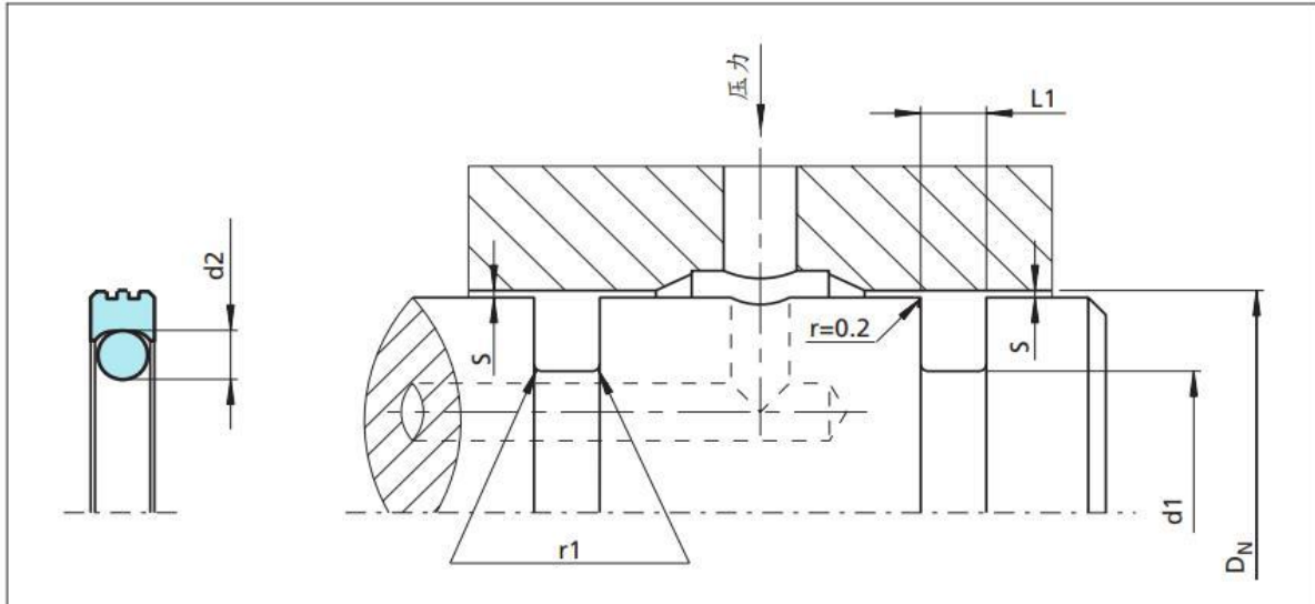
图 90 安装图
