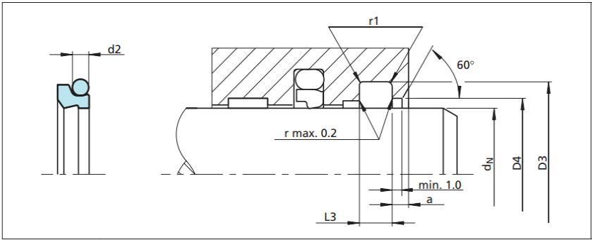
图37 安装图
